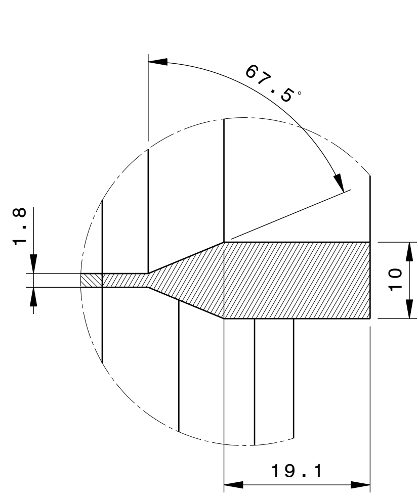
Detail D Scale: 2:1
