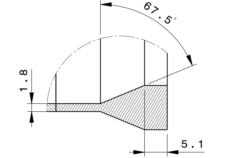
Detail E Scale: 2:1
