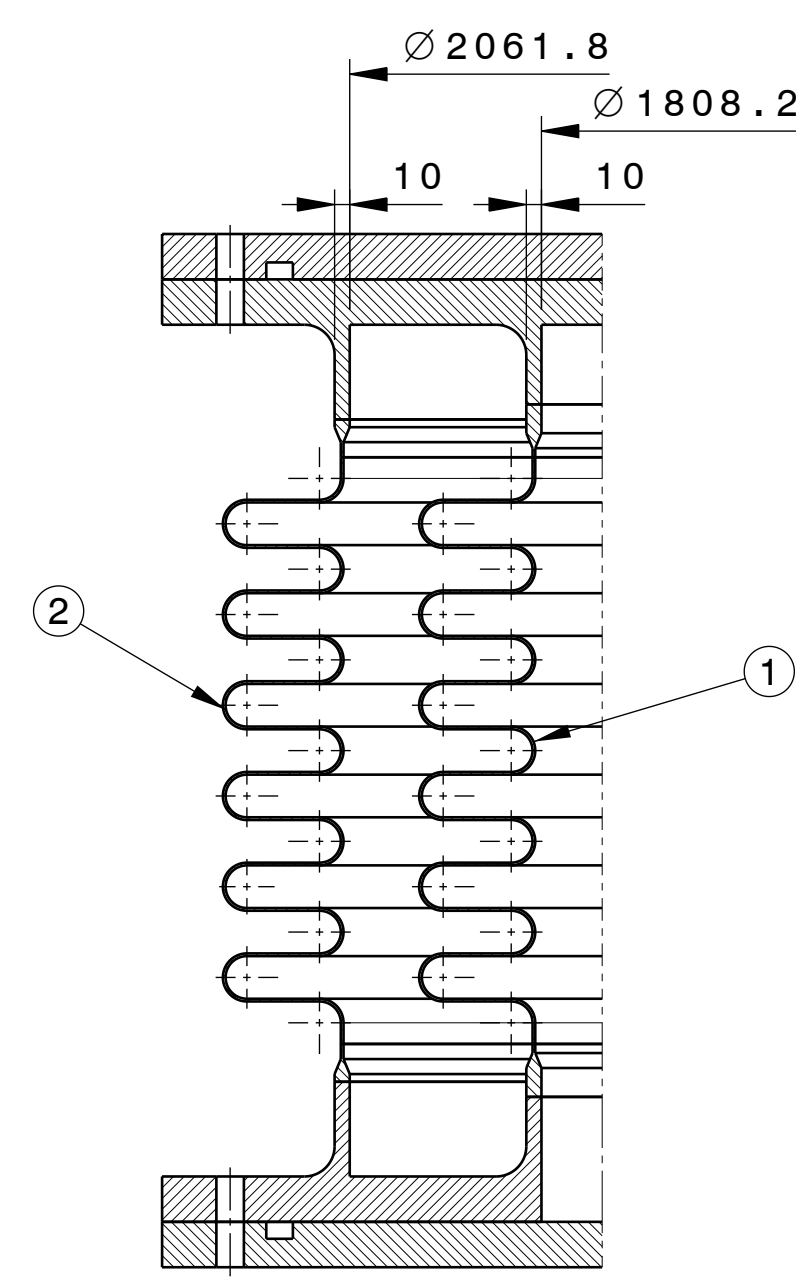
Detail D Scale: 1:5
