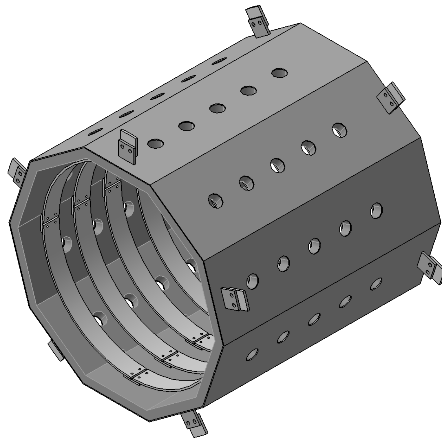
Isometric view Scale: 1:10
