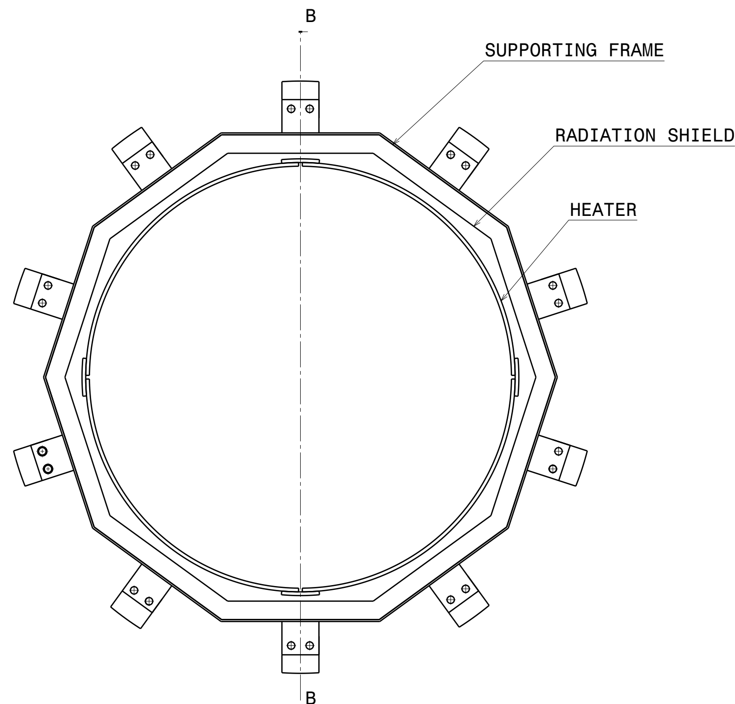
Front view Scale: 1:10
