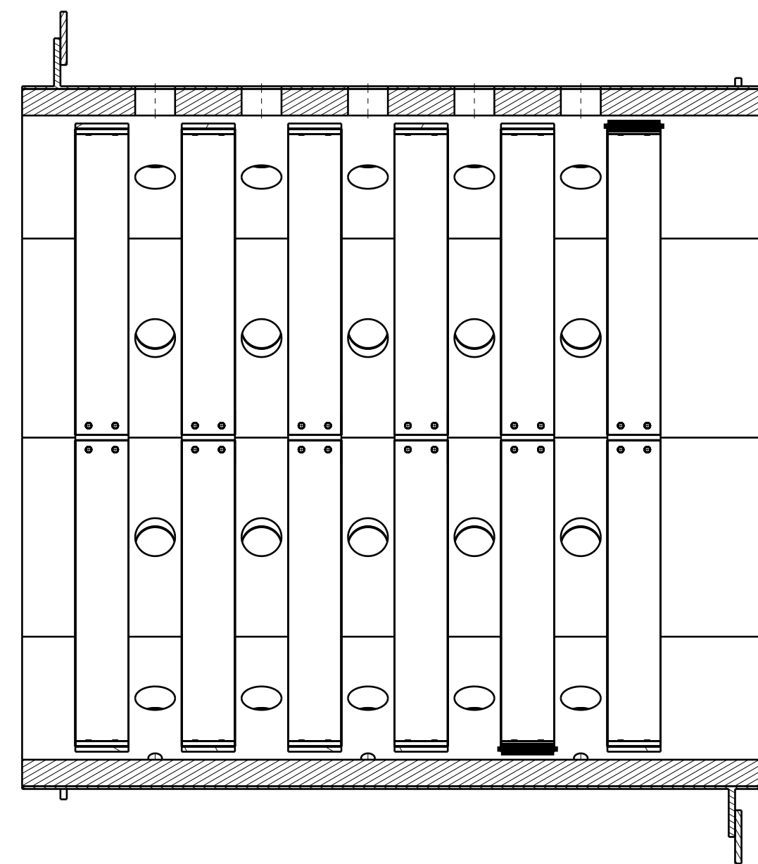
Section view B-B Scale: 1:10
