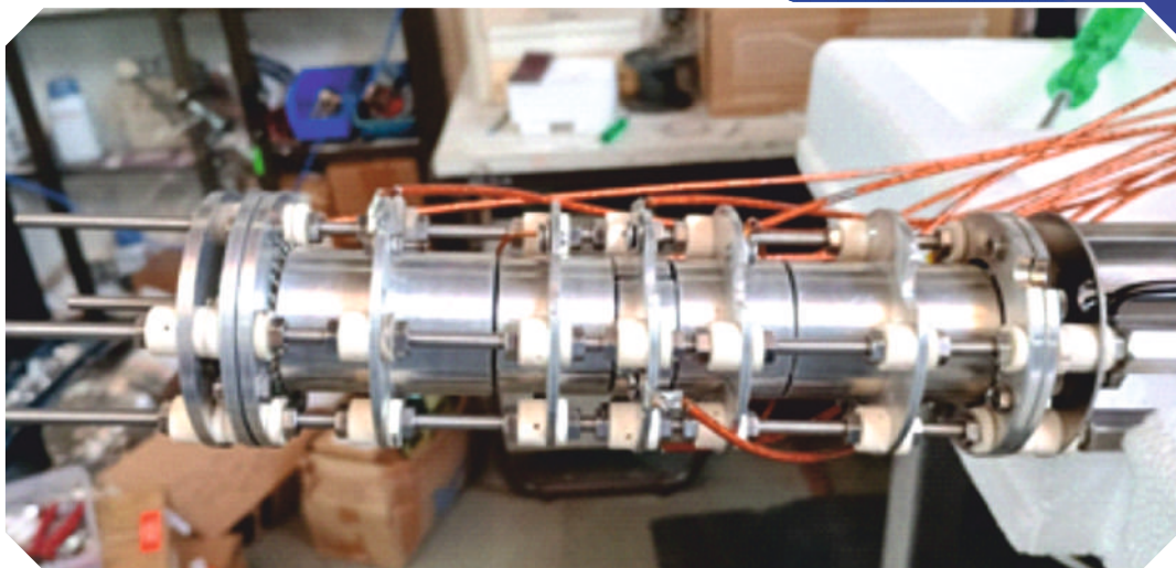
पाँच संकेन्द्रित बेलनाकार रिंग इलेक्ट्रोड, ग्रिड और फिलामेंट से निर्मित रेखीय बेलनाकार पेनिंग-माल्मबर्ग ट्रैप Linear cylindrical Penning – Malmberg Trap made up of five concentric cylindrical ring electrodes, grids and filament
